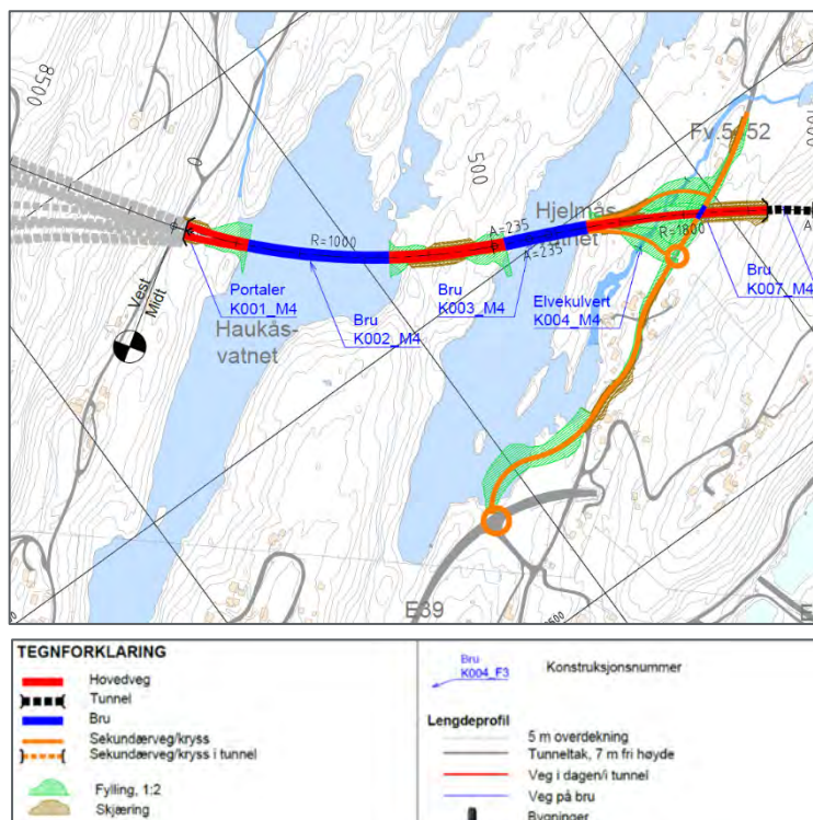
Figur 3-1. Det er i alternativ M4 ikkje planlagt fylling i sørenden av Hjelmåsvatnet. Utlaupe frå Hjelmåsvatnet skal gå i ny kulvert gjennom fylling nedstraums utlaupet (grønt areal), og vidare gjennom eksisterande kulvert under fv. 5452.
