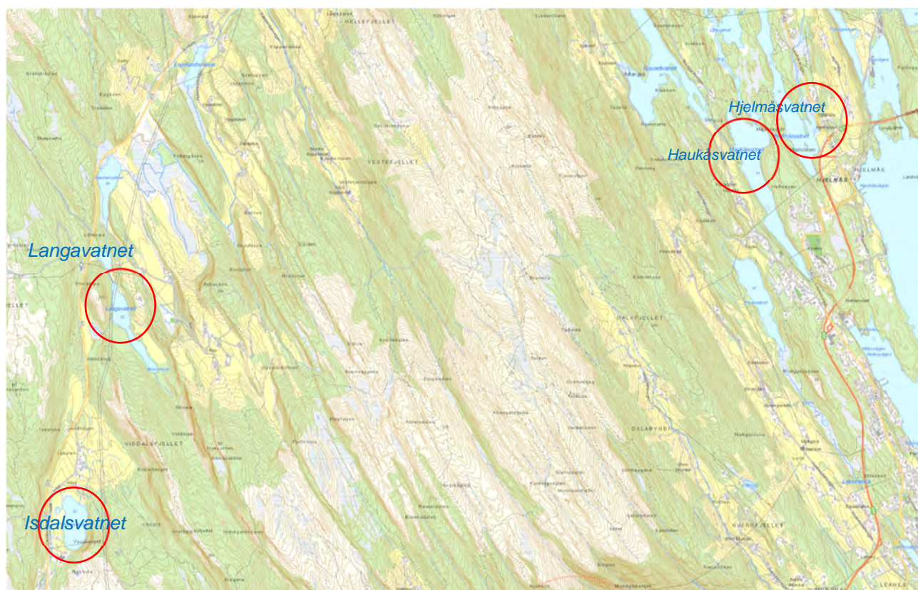
Figur 1-1 Kart som viser dei planlagde krysningane med nye E39 i dei ulike alternativa / områder kor det er gjort utrekningar av flaumvassføring og vasslinjeutrekningar.
