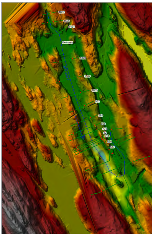
Figur 3-4 HEC-RAS 1D modellen nytta for Hjelmsvatnet.
